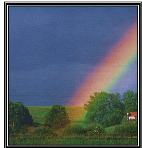
(Lichtbrechung in der Atmosphäre - Regenbogen)
