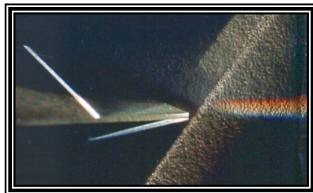
(Lichtbrechung durch ein Prisma)
